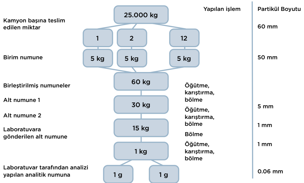
Şekil 3. Kilin karbonat içeriğinin tayini için örnek bir örnekleme planı akış şeması
